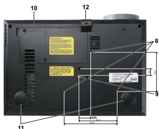
底面図
